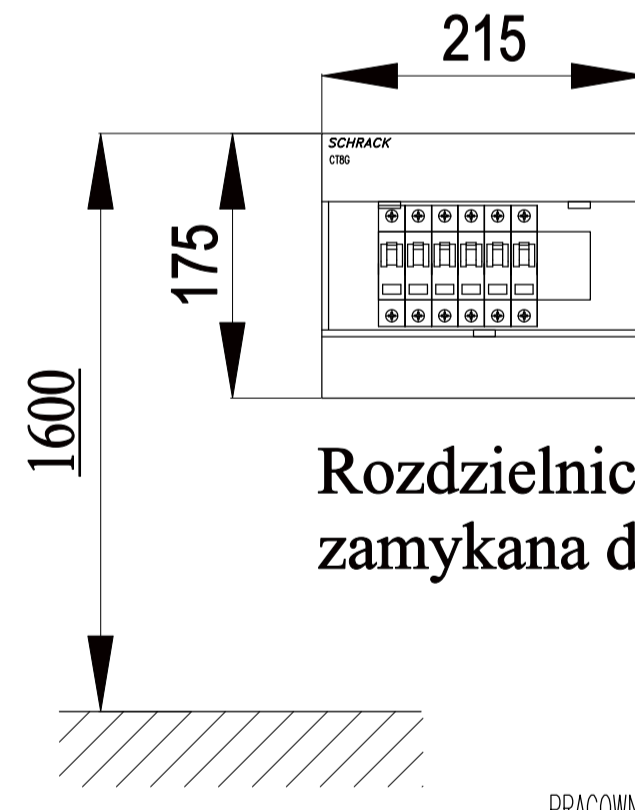
Tablica sterująca oświetleniem TR2 Widok. Skala 1-10
