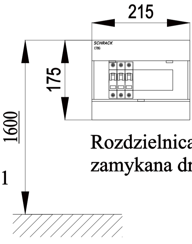
Tablica sterująca oświetleniem TR1 Widok. Skala 1-10
