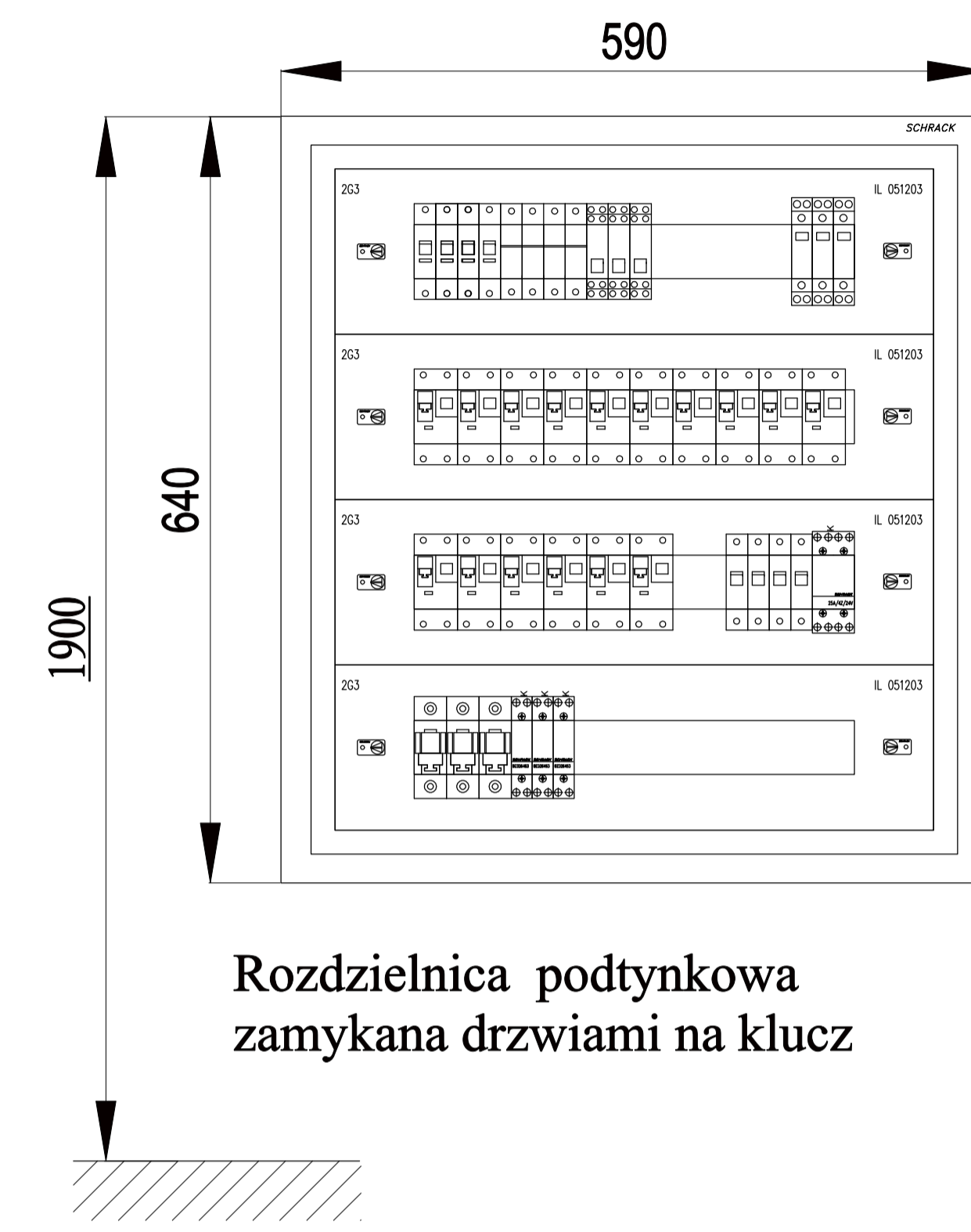
Tablica rozdzielcza T12 Widok. Skala 1-10
