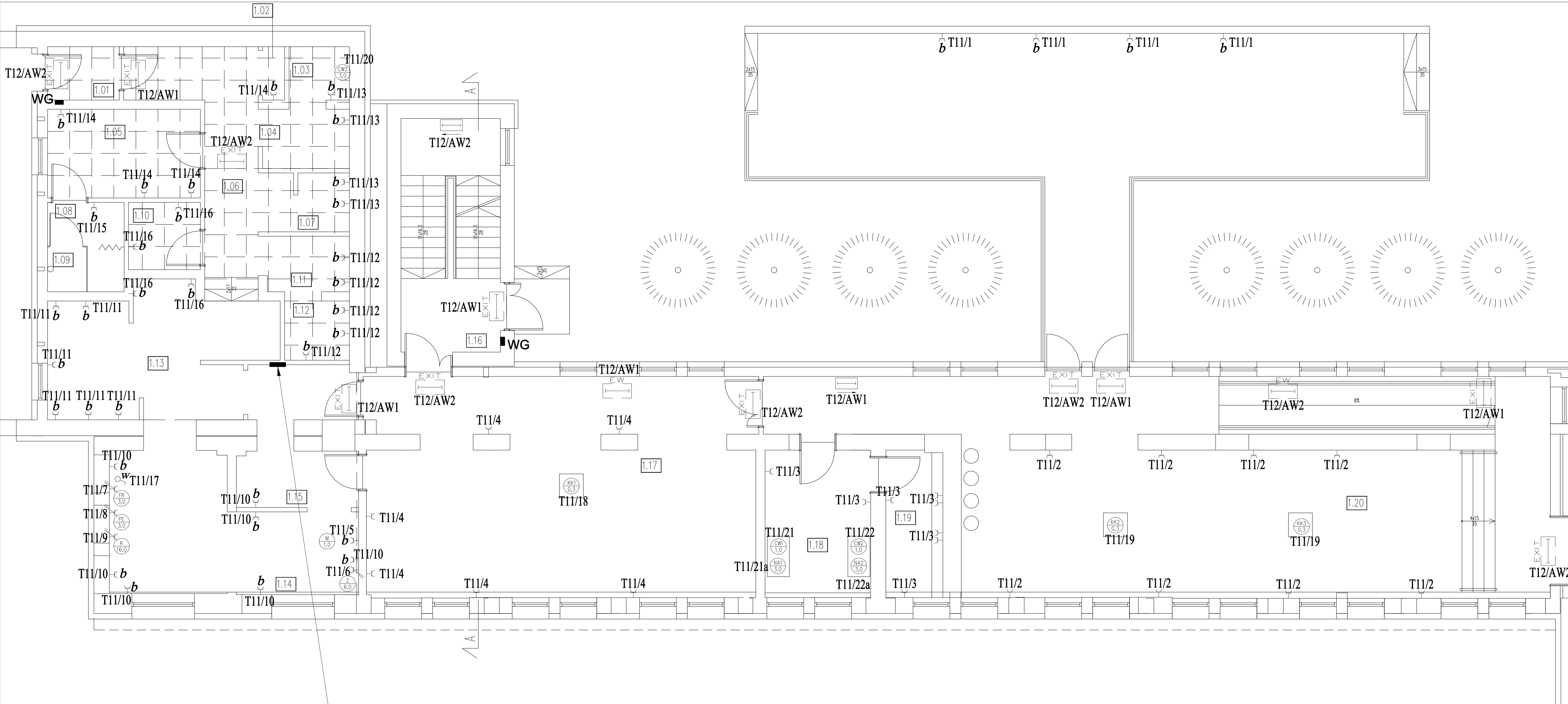
Tablica rozdzielcza T11 - rys. E-11
